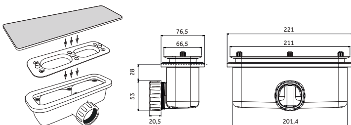
Piletta di scarico Side Plus
