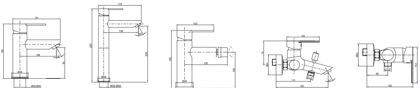
LAVABOCANNA ALTA Cartuccia ceramica 35 mm cold start Limitatore di portata ecologico 6 L/min Flessibili 3/8" NCE
